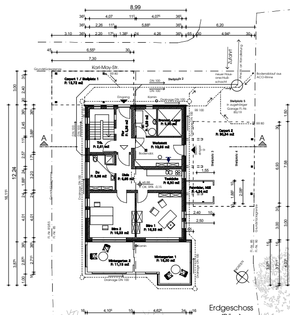
Erdgeschoss (Büro)
