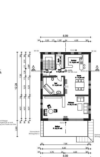
Obergeschoss (Wohnung)
