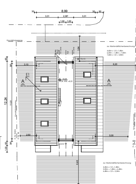
Spitzboden
