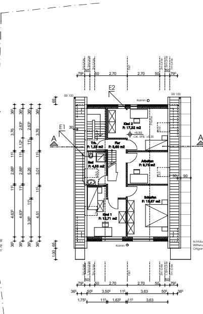
Dachgeschoss (Wohnung)
